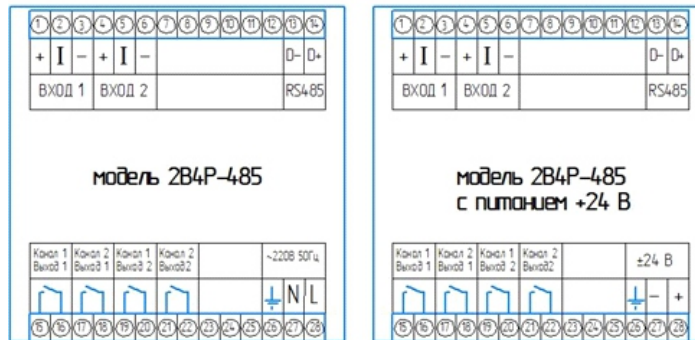
Схемы подключения датчиков
