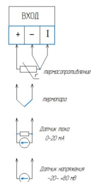
Схема подключения датчиков
