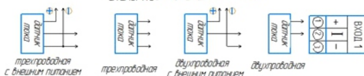
Схемы подключения датчиков
