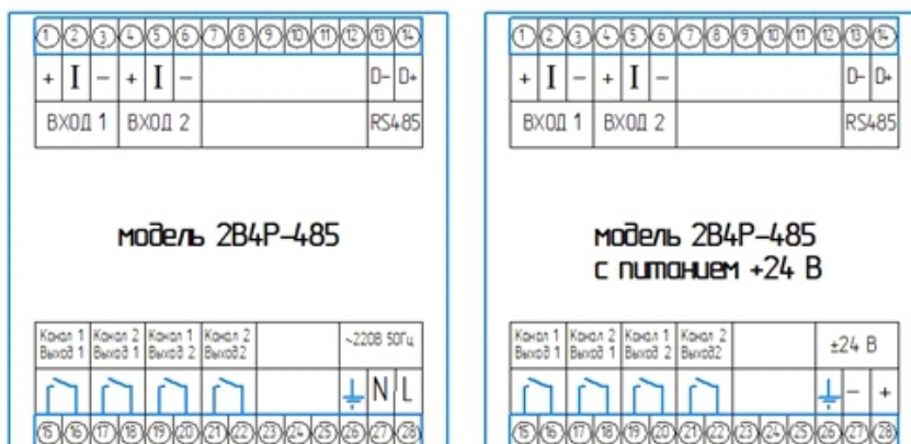
Схема расположения и состав выходов приборов ИСД322
