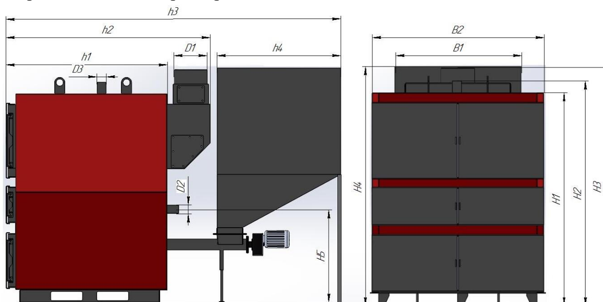
Чертеж для таблицы размеров ЭКО МАХDUO
